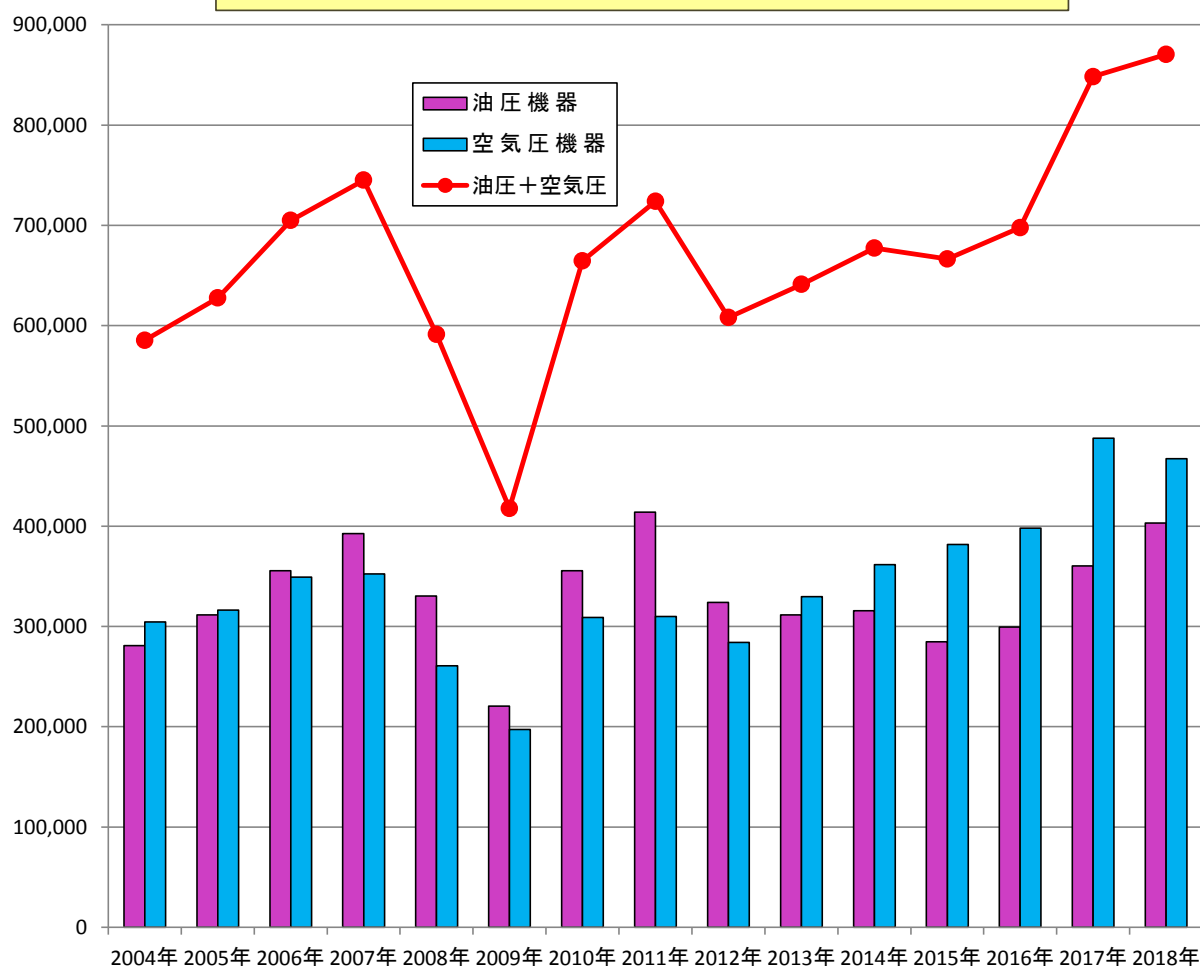
油空圧機器 出荷実績推移グラフ【年度】
